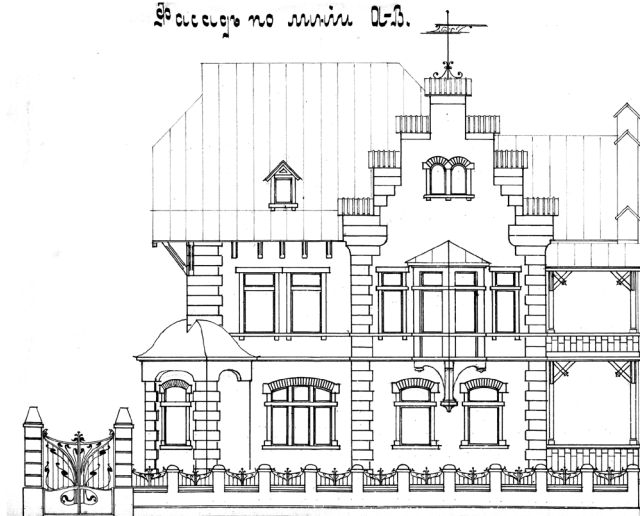
Рис. 5. Проект на постройку каменного двухэтажного дома А. Ю. Левицкого на Владимирской улице в первой части г. Вятки. 1909 г. Арх. Э. К. Нюквист. Кировский областной краеведческий музей им. П. В. Алабина
